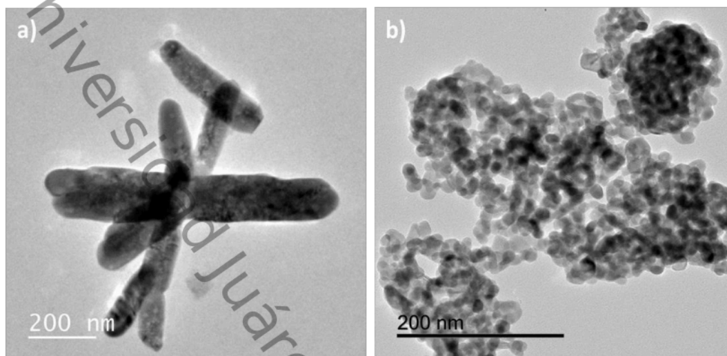
Figura 36. Imágenes TEM de las partículas a) \text{ZnO} , b) \text{ZrO}_2 , a pH 9 y calcinadas a 500 °C.
