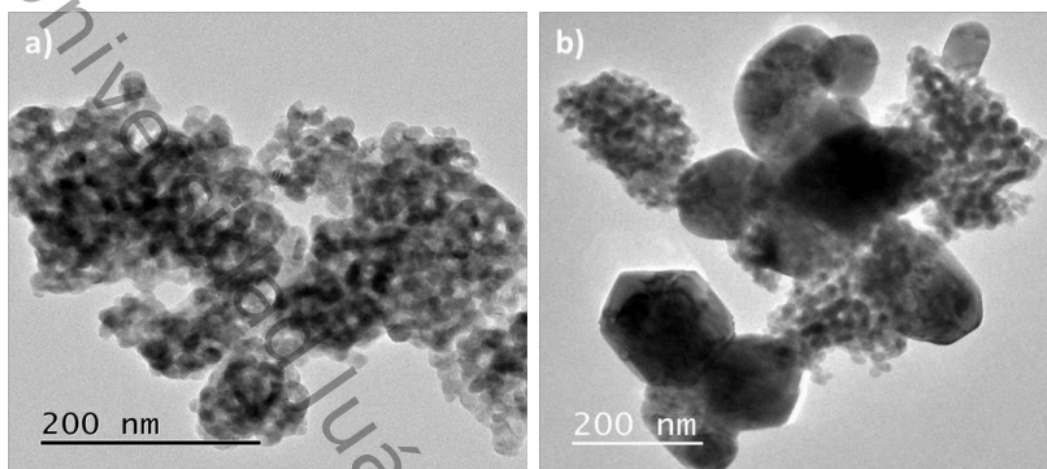
Figura 37. Imágenes TEM de las partículas a) \text{ZnO-ZrO}_2 con 13% mol \text{ZnO} , b) \text{ZnO-ZrO}_2 con 75% mol \text{ZnO} , a pH 9 y calcinadas a 500 °C.
