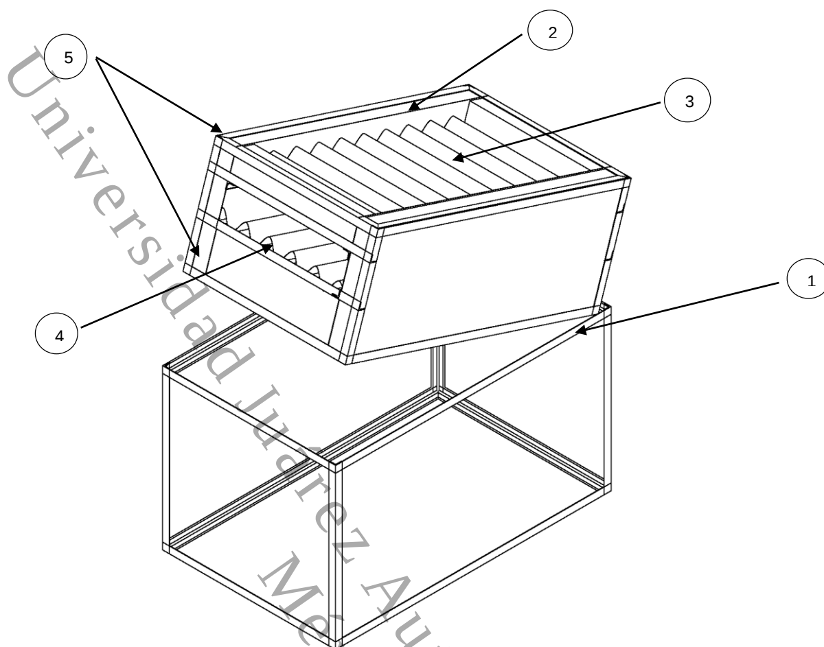
Figura 4.2. Esquema de las partes del colector solar: 1) soporte; 2) placa traslúcida; 3) placa absorbidora; 4) placa de fondo; 5) aislante térmico.
