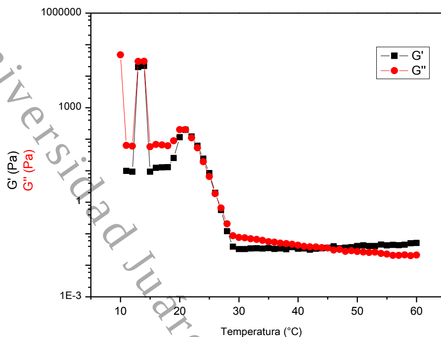
Figura 40. Módulo elástico ( G' ) y módulo viscoso ( G'' ) en función de la temperatura del sistema DeSan/agua al 10 % en peso.
